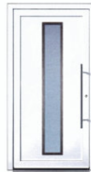
THERMO 1 U_D -Wert 1,23 Farbe: Verkehrsweiss Mindestmaß: 800 x 1.990 mm
